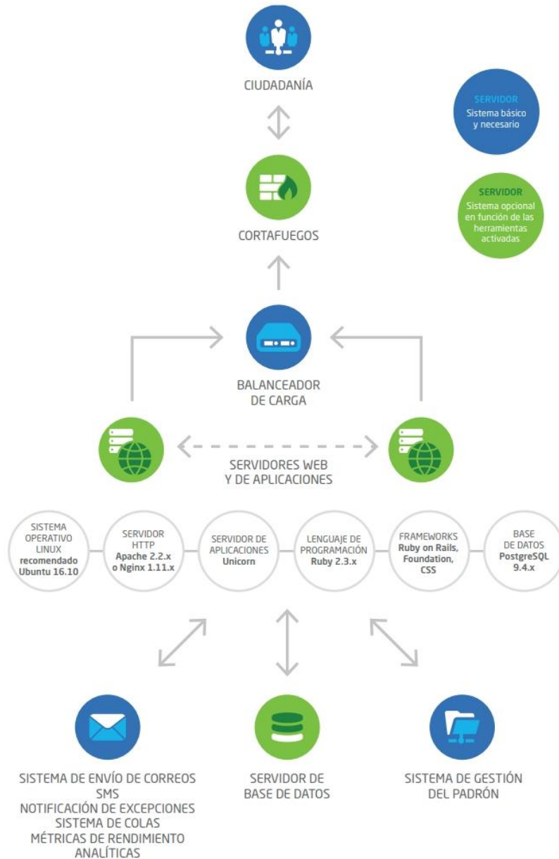
Arquitectura 13 necessària per la posada en marxa de Decidim.
